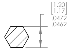
SECTION A-A SCALE 8 : 1
